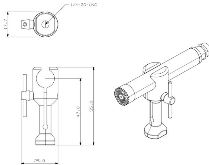
LH 006 1/2 尺寸图
